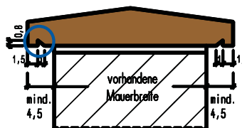
Mauerabdeckung Pultdach
