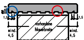
Mauerabdeckung flach-strukturiert
